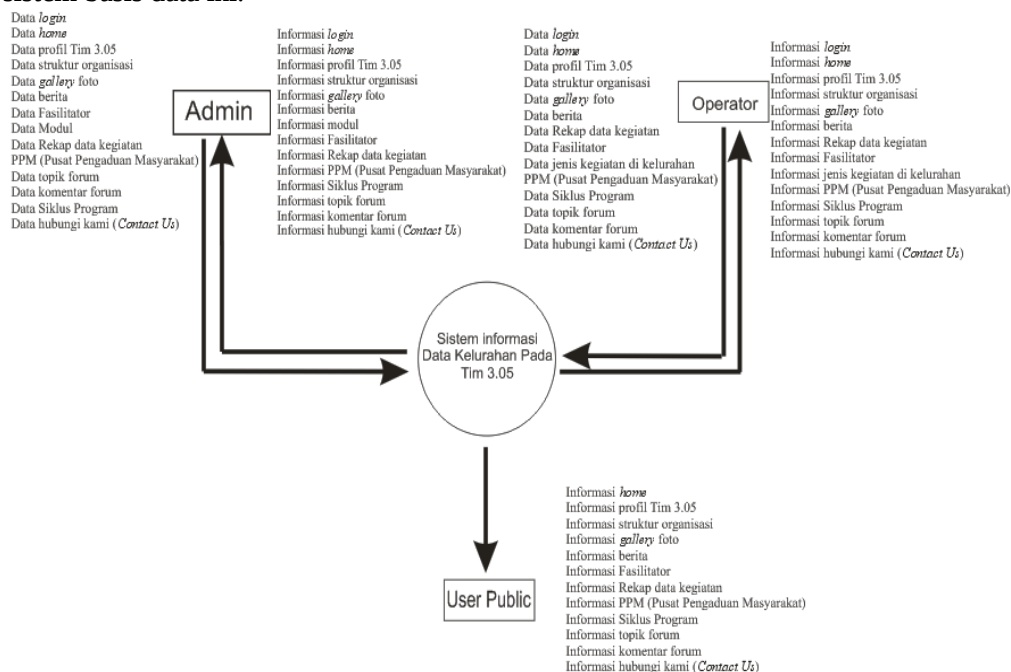
Gambar 1: Diagram Konteks
